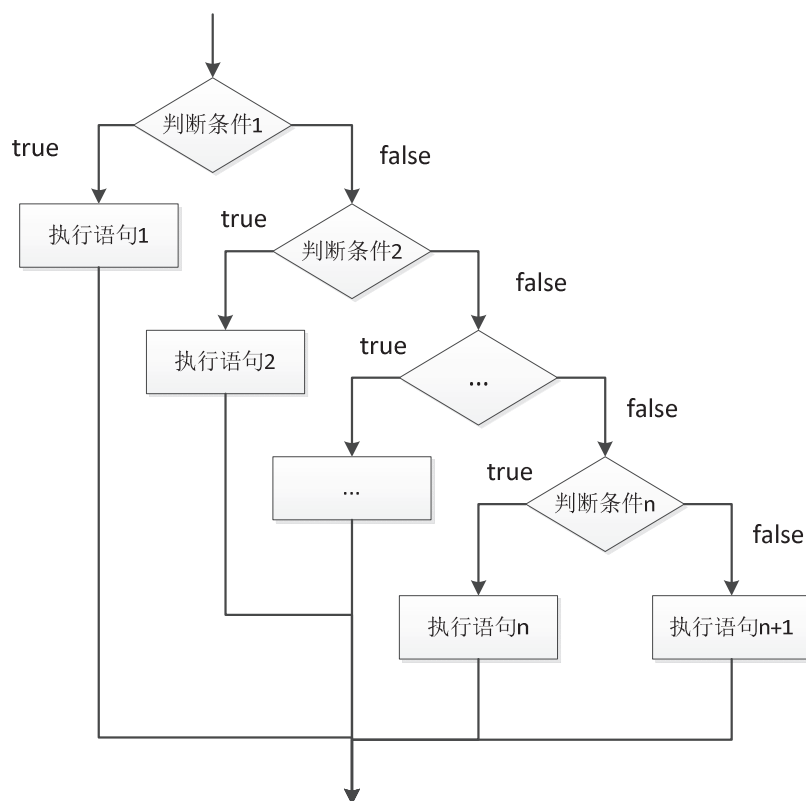
图7-17 多向判断语句执行流程
