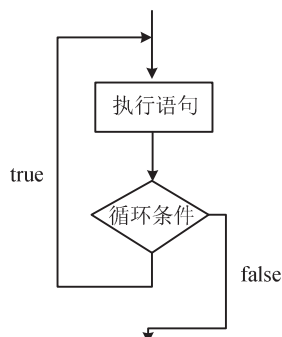
图7-22 do...while循环语句的执行流程
