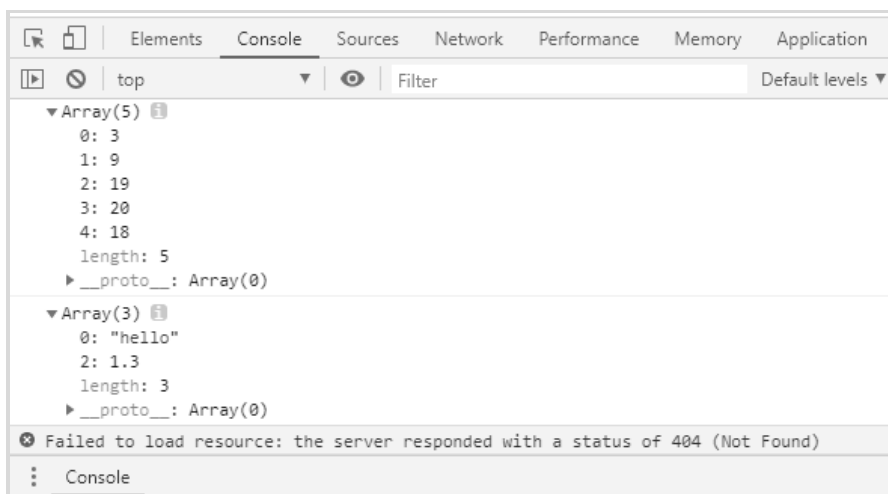
图8-11 未定义元素控制台输出结果
